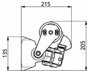
Ansicht Wandmontage
