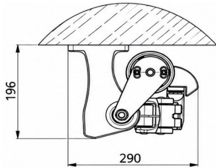
Ansicht Deckenmontage
