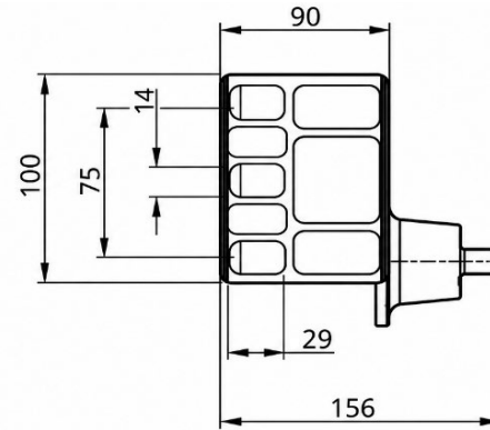
Konsole Deckenmontage
