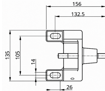
Konsole Wandmontage
