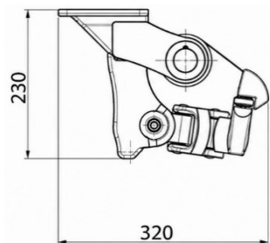
Anschauung Deckenmontage
