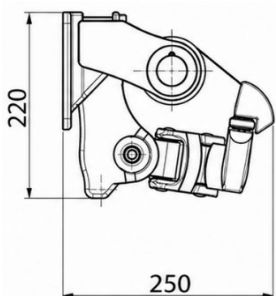
Anschauung Wandmontage
